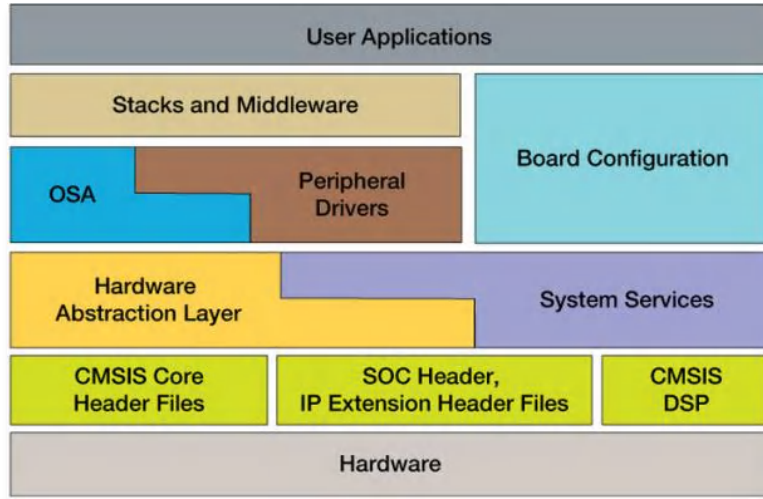
图 79 KSDK的总体结构
