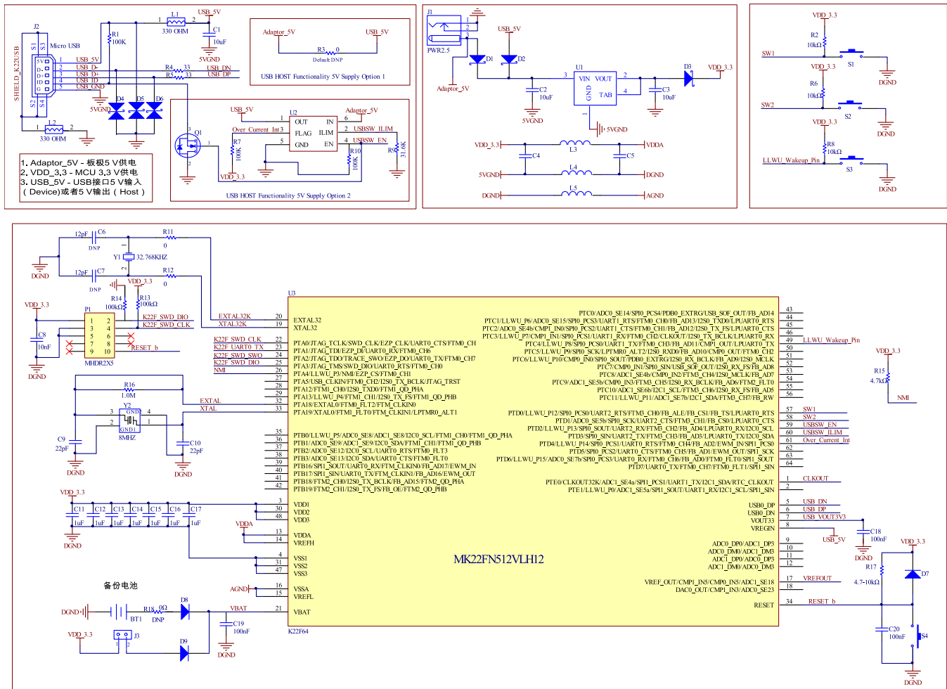
图 113 K22F 120M LQFP-64pin 最小系统原理图
