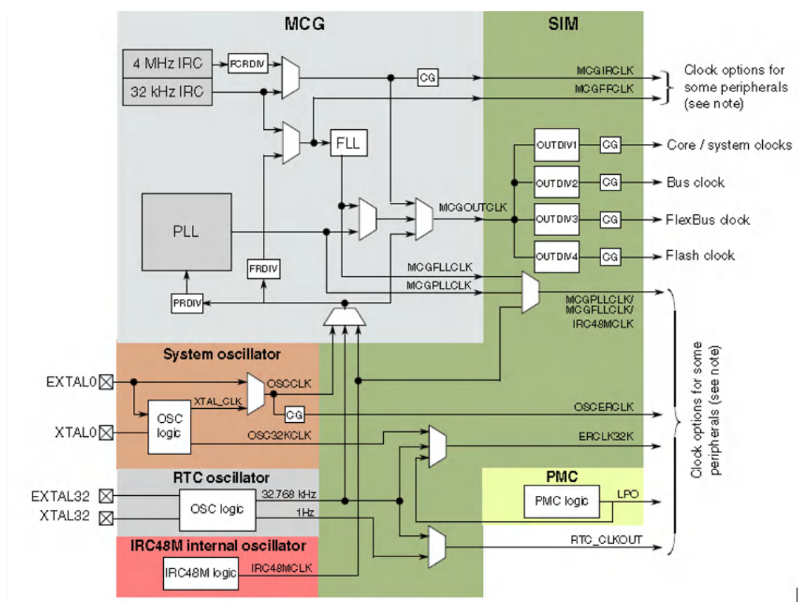
图 101 K22的系统时钟框图
