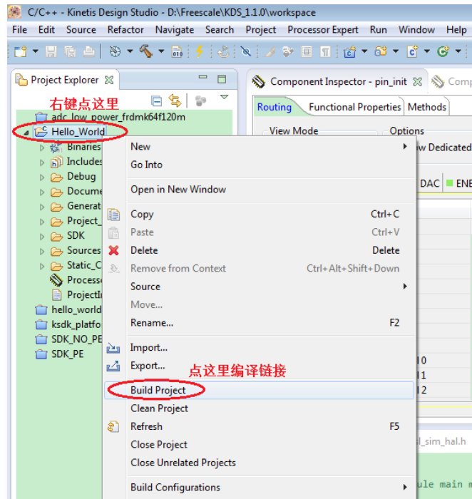
图 128 编译工程
